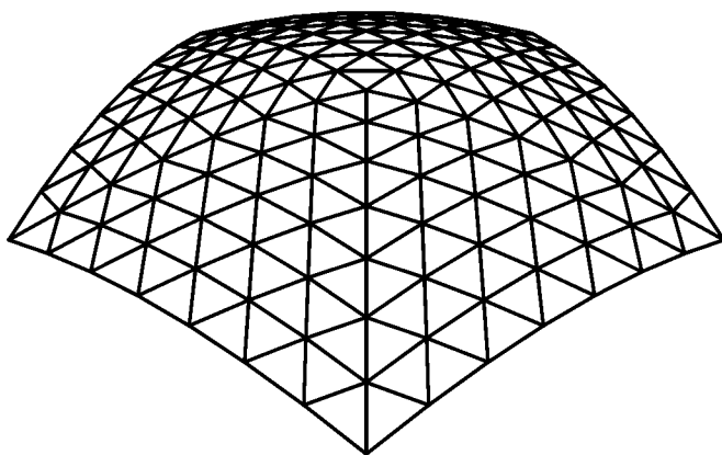
شکل ۱۵۳- گنبد قاجی نوانشی با نقش سه‌راهه و گوشه‌های درجا نگهداشته (حالت ۳ نوانش و یک نقطه مرکزی برآمده به کار رفته است)
