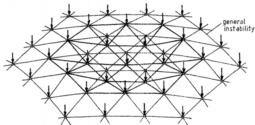
شکل پ-۴-۷ ناپایداری کلی
