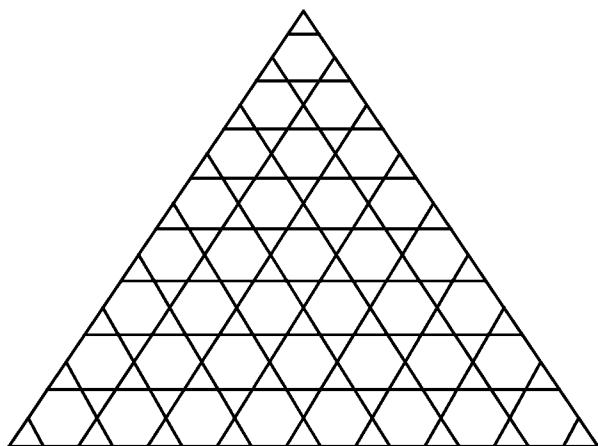
شکل ۱۵- شبکه مثلثی تک لایه با نقش سه راهه / شش بری
