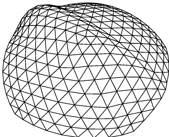
شکل ۱۹۰- شکل آزاد: گنبد پخش‌شده ژئودزیک فرازیده (یک فرازش استوانه‌ای با مقطع سهمی به کار رفته است)
