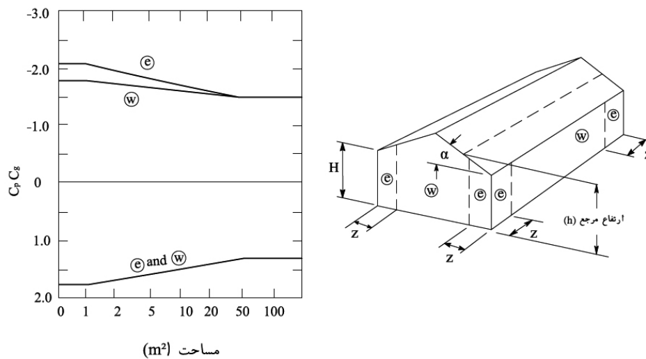
شکل ۹-۳- حداکثر ضریب خارجی C_g C_p در دیوارهای تک برای طراحی اجزای نمای ساختمان‌ها
