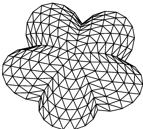
شکل ۱۱۴- گنبد اسکالپ با کد ۱، برآمدگی ۸ و پیش آمدگی ۱۵
