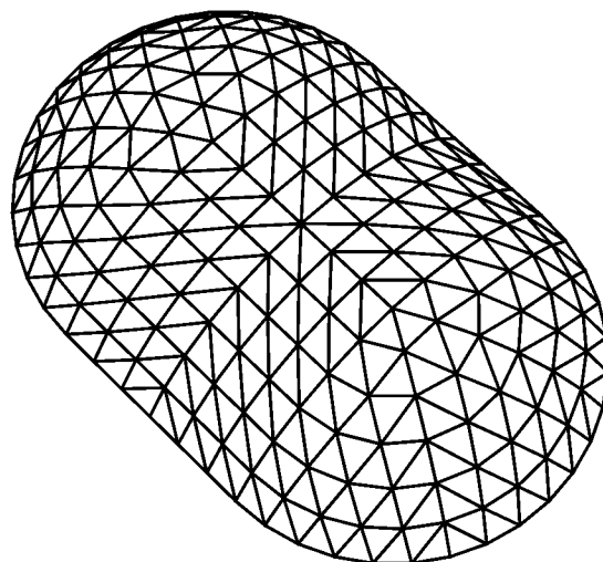
شکل ۱۶۱- چلیک-گنبد
