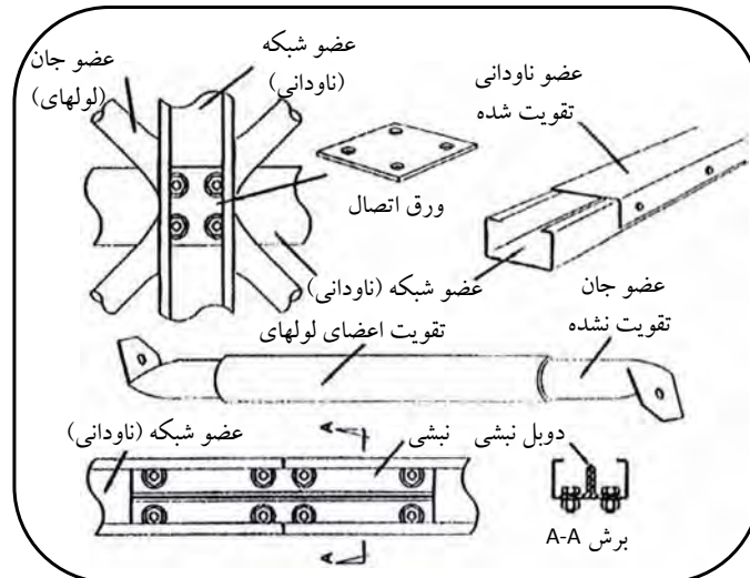
شکل (۴۵) : صفحات تقویت کننده در سیستم HARLEY
