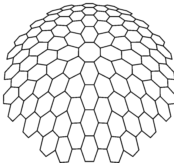
شکل ۱۳۷- گنبد قاچی فرازشی (سهموی) با نقش لانه زنبوری
