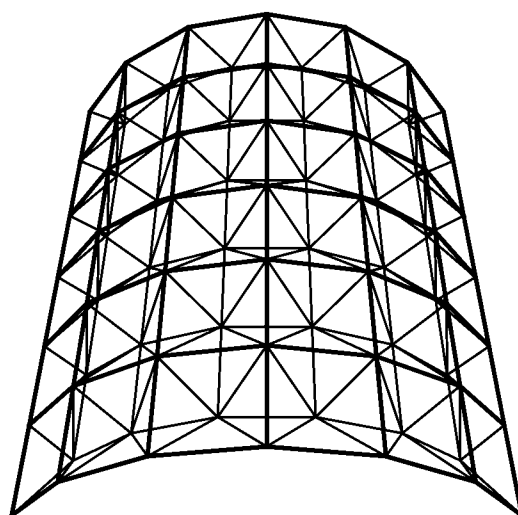
شکل ۷۱- چلیک دو لایه با نقش دوراھه روی دوراھه
