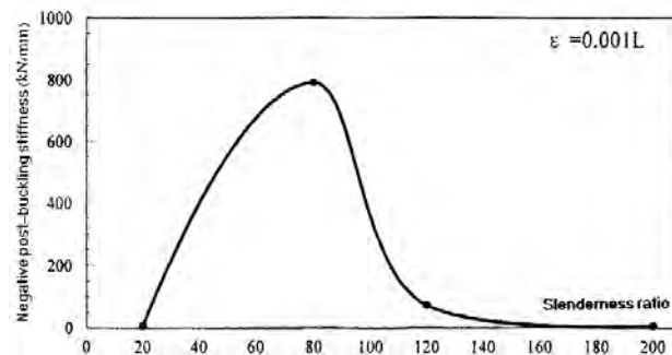
شکل پ - ۵-۴- نمودار تقریبی تغییرات سختی منفی پس کمانشی - نسبت لاغری به ازای ناکامی اولیه \varepsilon = 0.001L
