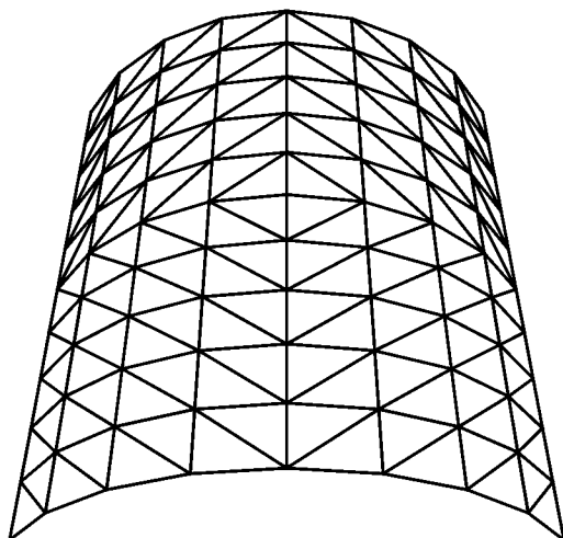
شکل ۶۹- چلیک دوراوه با هموندهای قطری اضافی
