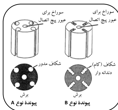
شکل ۶-۹: نمونه ای از اتصال کام و زبانه ای
