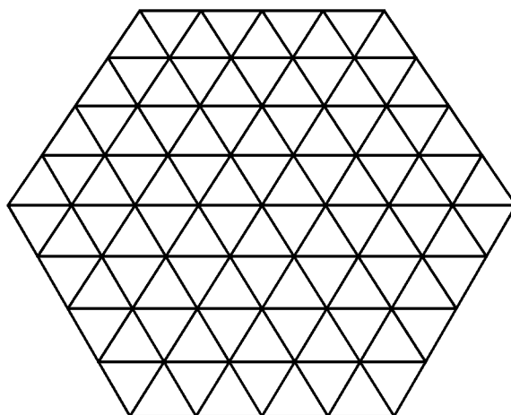
شکل ۱۴- شبکه مثلثی تک لایه با نقش سه راهه و گوشه های بریده
