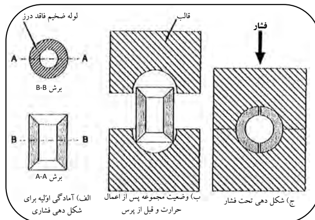
شکل (۱۰): روند تولید پیونده UNITRUSS
