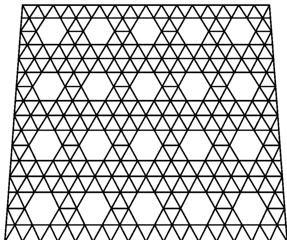
شکل ۱۰- شبکه تک لایه با نقش سه راهه/شش بوی
