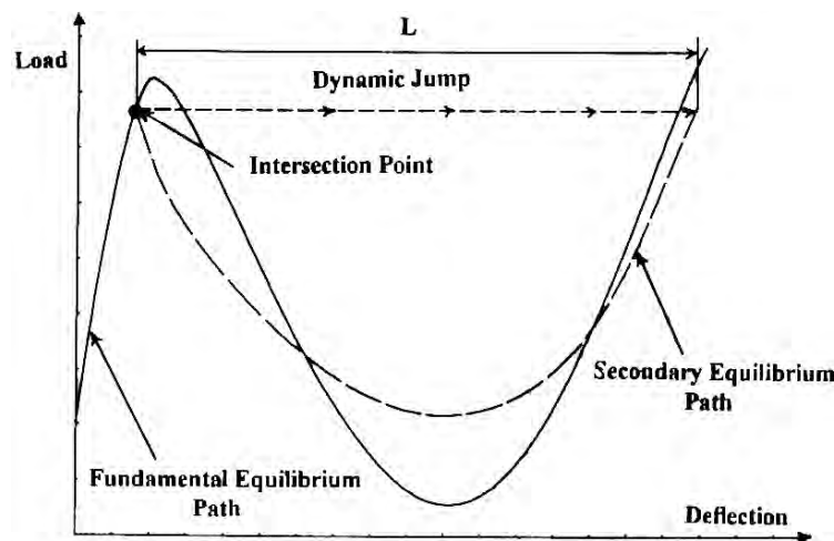
شکل پ-۴-۵-۲- فروجهش دینامیکی در ناپایداری نقطه دوشاخگی متقارن ناپایدار
