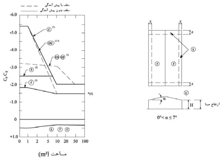
شکل ۳-۱۰- حد/کثر ضریب خارجی C_{pe}C_g در سقف های با شیب کمتر از ۷ درجه برای طراحی اجزای سازه ای و نما
