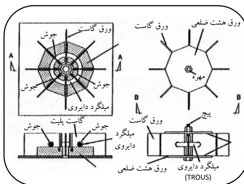
مطابق شکل ۲۹، سیستم پیونده صفحه‌ای Torus Gesto، از دو صفحه هشت ضلعی و هشت ورق فولادی مستطیلی، میلگرد، پیچ و مهره تشکیل شده است. ابتدا ورق‌های فولادی به صفحه تحتانی جوش شده و میلگردی دایروی از مابین سوراخ‌های آنها عبور داده می‌شود که به آنها جوش می‌گردد. بعد از جوش کاری، صفحه فوقانی به قطعات مزبور پیچ می‌شود. در این سیستم، اعضای سازه‌ای می‌توانند با جوش کاری یا پیچ به پیونده متصل گردند.
