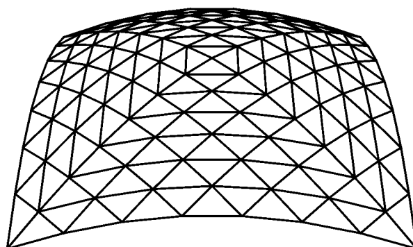
شکل ۱۵۲- گنبد قاجی نوانشی با نقش سه‌راهه و گوشه‌های درجانه‌گذاشته (حالت ۳ نوانش و یک نقطه مرکزی برآمده به کار رفته است)
