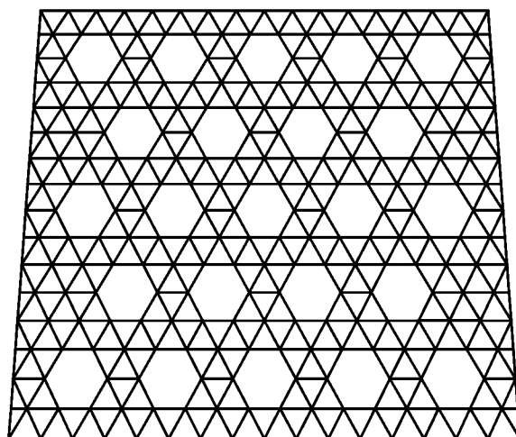
شکل ۱۱- شبکه تک لایه با نقش سه راهه/شش بوی
