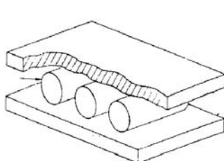
شکل ۴-۲: تکیه‌گاه چند غلتکی
