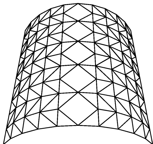
شکل ۷۰- چلیک دوراھه با هموندهای قطری اضافی
