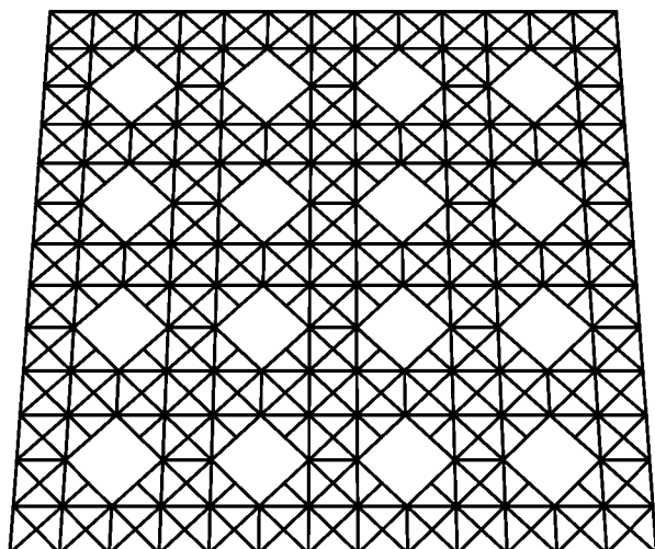
شکل ۳۳- شبکه تک لایه با نقش چهار راهه و چشمه های باز
