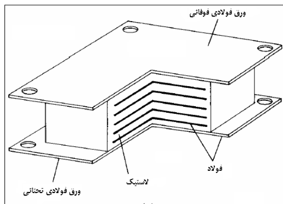
شکل ۶-۶- جداگر لاستیکی طبیعی و مصنوعی با میرایی کم
