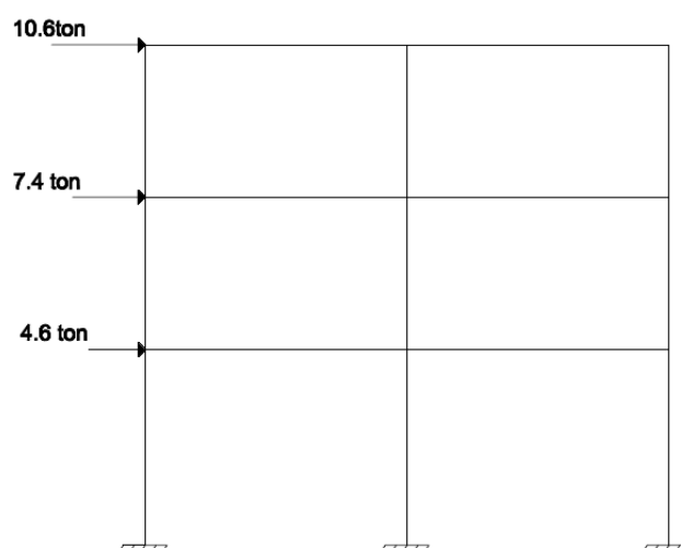
شکل ۳۲-۶ - توزیع نیروی زلزله در ارتفاع
