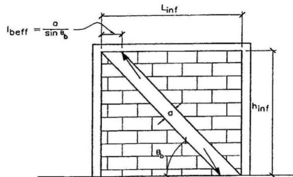
شکل مثال ۴-۲-ع- نیروی برشی وارد به تیر از طرف پانل میانقاب
