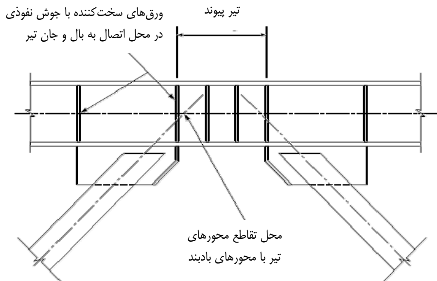
شکل ۴-۱۳- جزئیات تیر پیوند و مکانیسم تسلیم در قاب‌های مهاربندی شده بوسیله مهاربدهای واگرا
