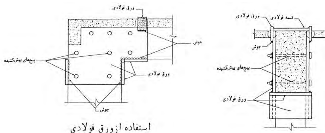
شکل ۲-۶-۲۴ روش‌های بهسازی اتصالات کناری
