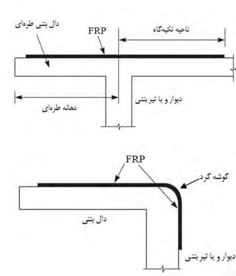
شکل ۲-۳-۱۴- سایر روش‌های تأمین طول مهاري با امتداد FRP روی دال‌ها
