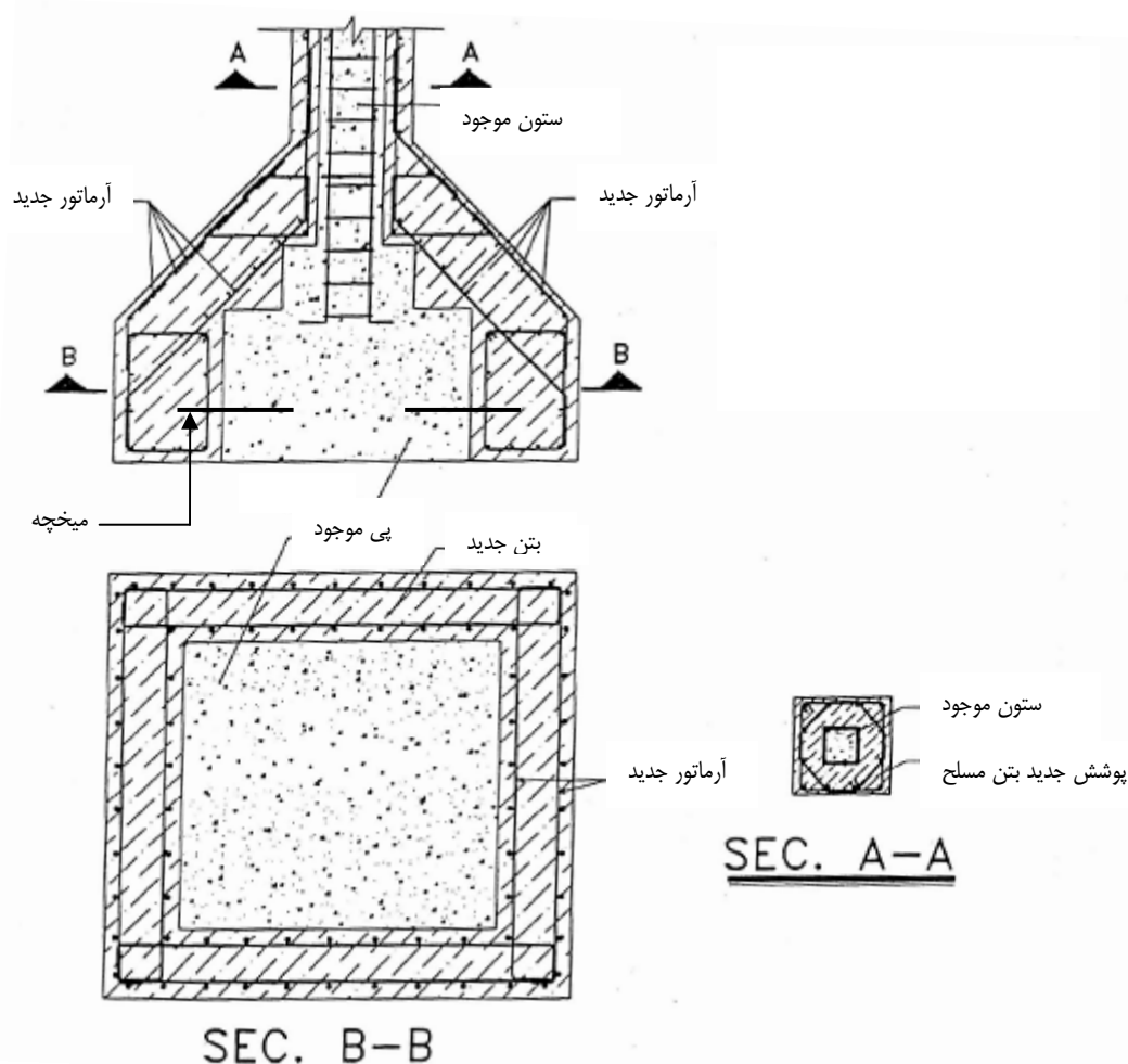
شکل ۲-۲-۱- افزایش ابعاد شالوده و ستون متصل به آن
