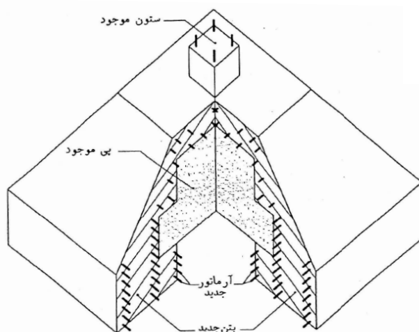
شکل ۲-۲-۲- بهسازی شالوده بوسیله افزایش ابعاد هندسی
