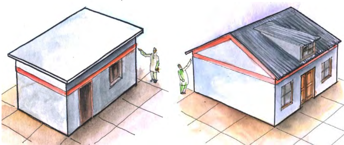
شکل ۹-۷ موقعیت تسمه‌های افقی لرزه‌ای
