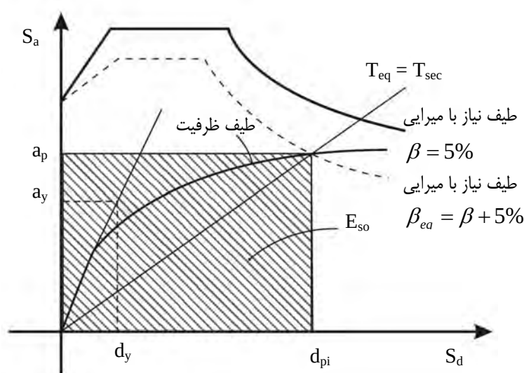
شکل ۵-۱- مشخص کردن نقطه عملکرد و جابجایی هدف
