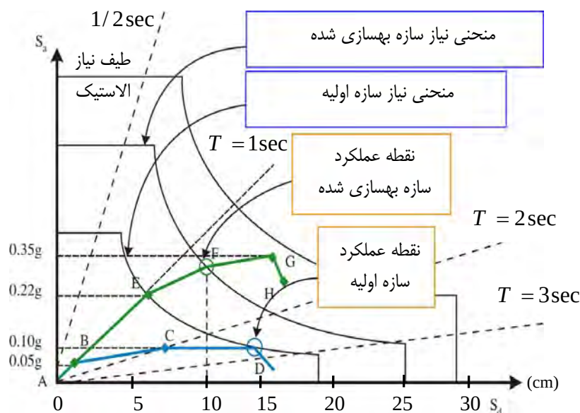
شکل ۱-۱- تاثیر افزایش مقاومت سیستم در عملکرد لرزه‌ای سازه
