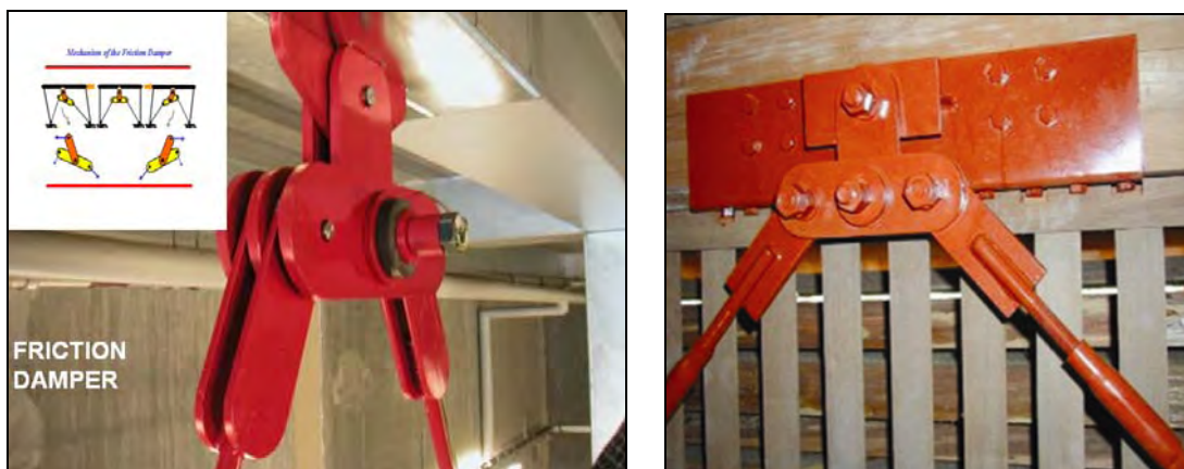
شکل ۵-۷ - استفاده از میراگرهای اصطکاکی چرخشی در مقاوم سازی
