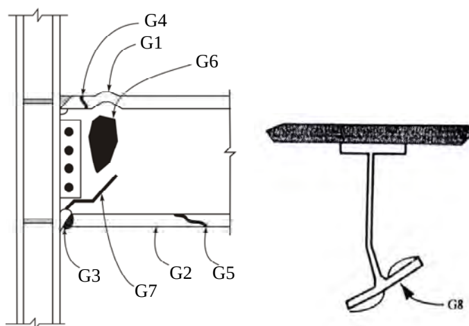
شکل ۳۳-۶-۲ خرابی در تیرها
