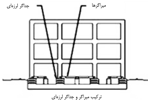
شکل ۷-۱۶- جزئیات تیپ سیستم میراگر ویسکوز
