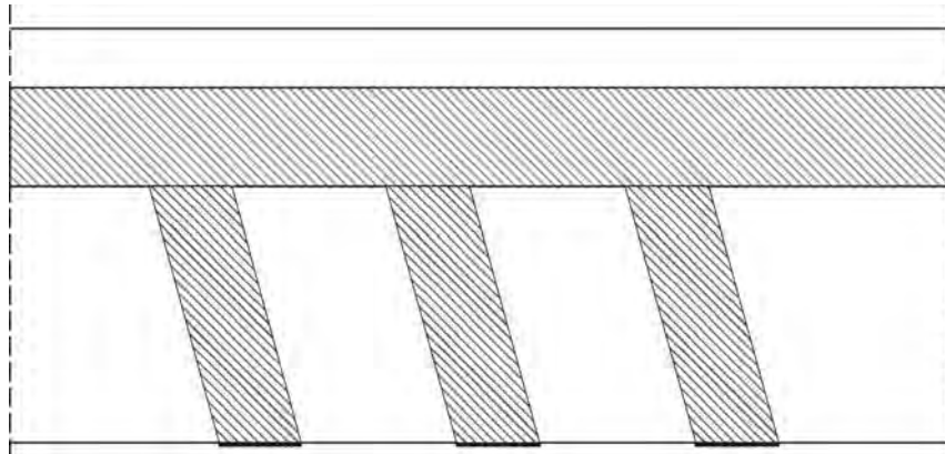
شکل ۲-۴-۱۳- نمایش از تقویت برشی
