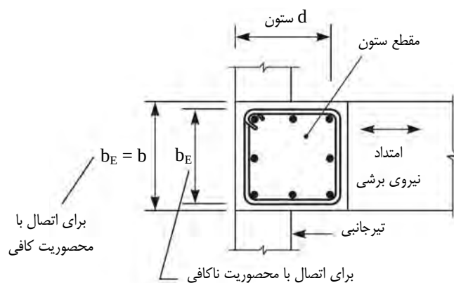
شکل ۲-۶-۱۴ هسته اتصال
