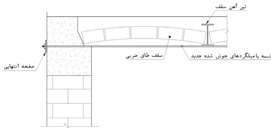
شکل ۸-۹ - بهسازی سقف با مهار پطاق
