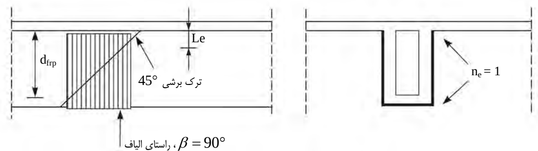
ب- رکابی‌های U شکل FRP
