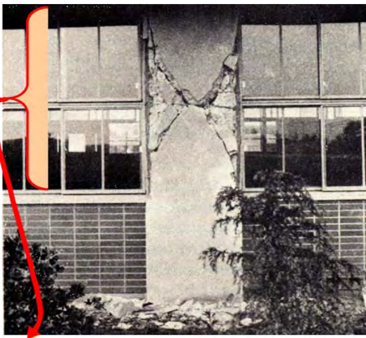
ستون کوتاه
