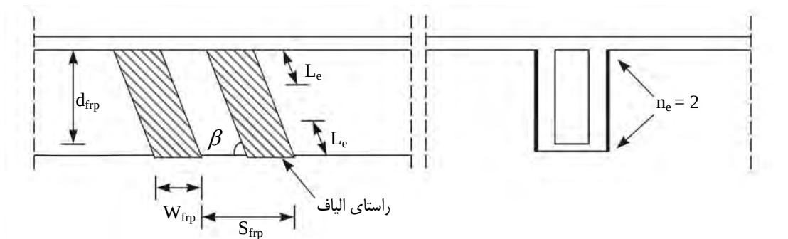
الف- تقویتی‌های برشی FRP بر وجوه جانبی
