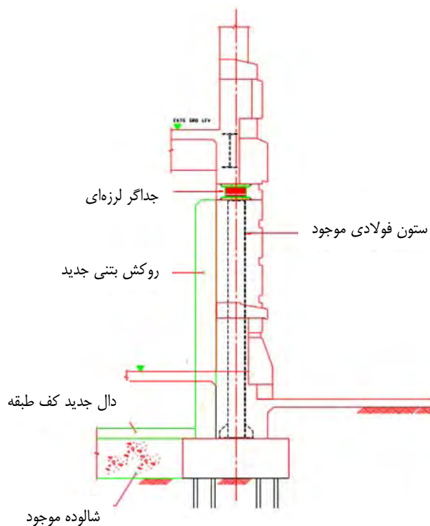
شکل ۶-۲۶ - جزئیات تیپ نصب جداگر در ستونهای فولادی
