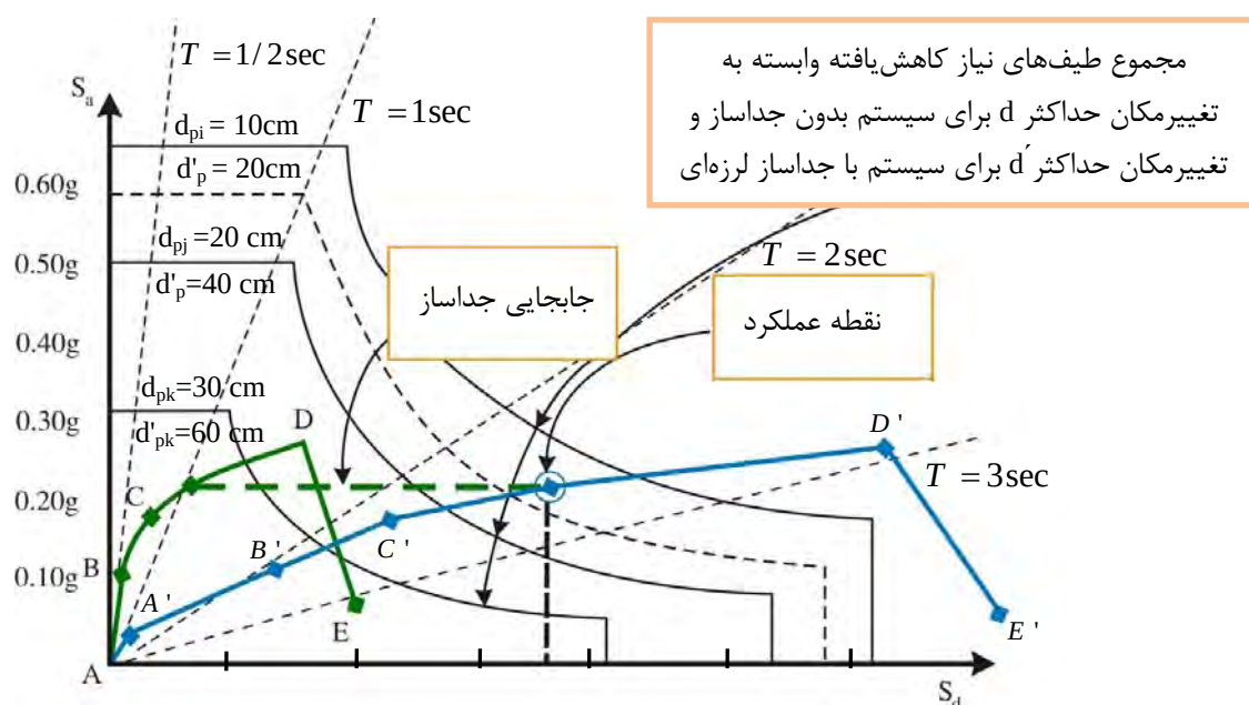
شکل ۱۳-۱ - تأثیرات استفاده از جداسازهای لرزه‌ای بر طیف نیاز و ظرفیت سازه
