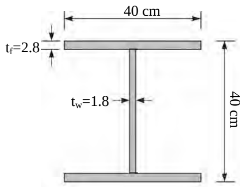
مقطع ستون
