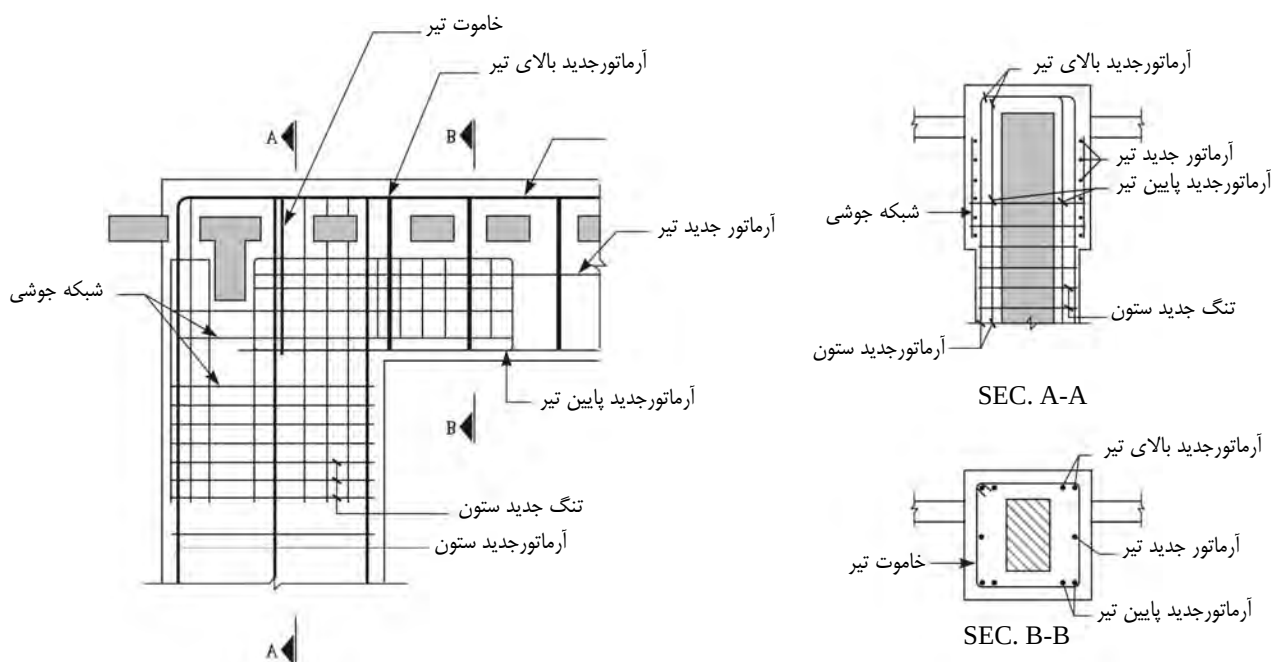
شکل ۲-۶-۲۳ اجرای روکش بتنی در اطراف اتصال خارجی
