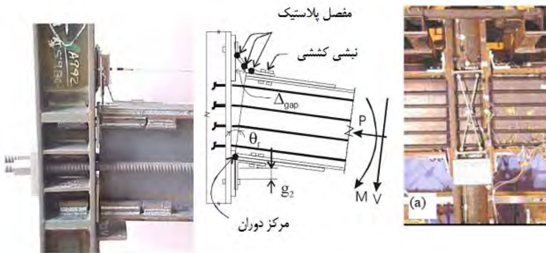
شکل ۴۶-۶-۲ مقاوم‌سازی اتصال با پیش‌تنیدگی خارجی بوسیله کابل کششی
