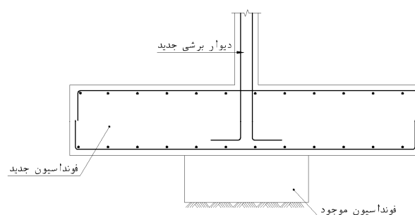
شکل ۸-۲۶ - پی جدید دیوار برشی
