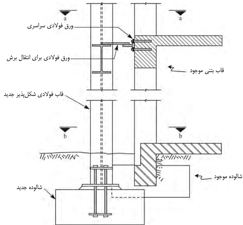
مقطع دیوار
