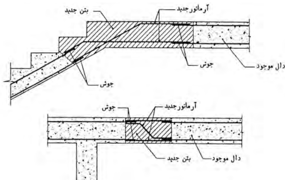
شکل ۲-۳-۱- تعمیر موضعی دال‌های کف و راه‌پله
