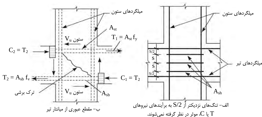
شکل ۱۳-۶-۲ نیروهای موجود در هسته اتصال [۱۹]
