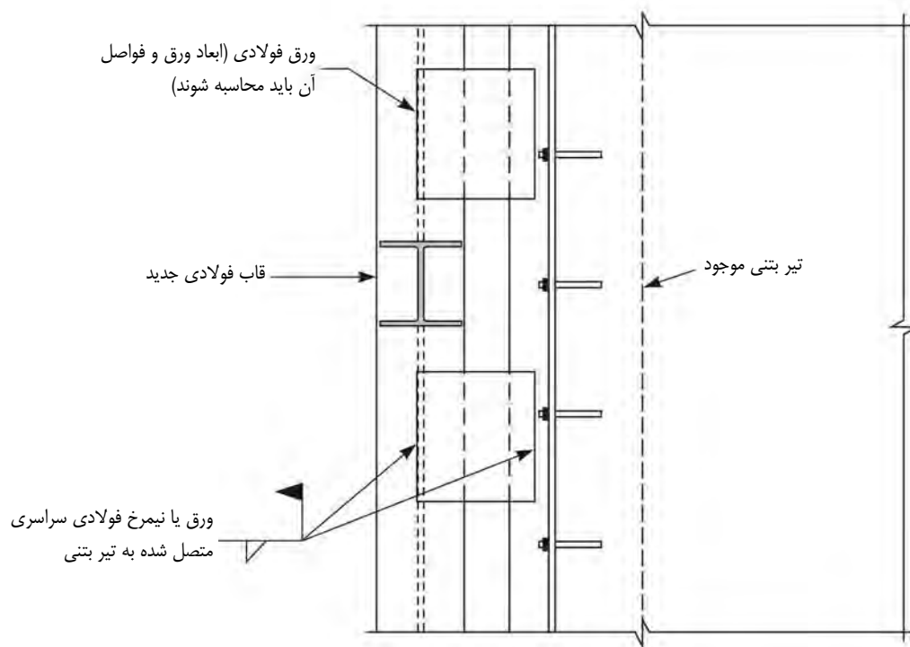
مقطع a-a
