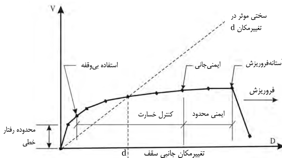
شکل ۲-۱- منحنی ظرفیت تیپ
