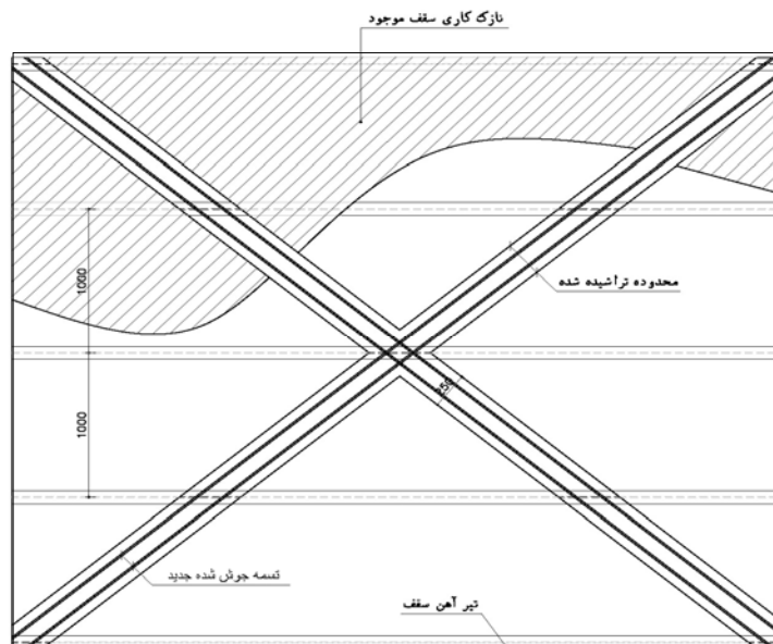
شکل مثال ۱-۸-ح- بهسازی سقف با تسمه فولادی
