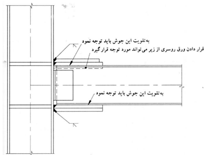
شکل ۴۱-۶-۲ تقویت اتصال با ورق زیرسری و روسری مضاعف
