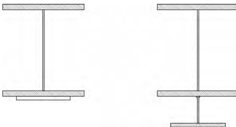
۲-۴-۲۱- تقویت با روکش فولادی
