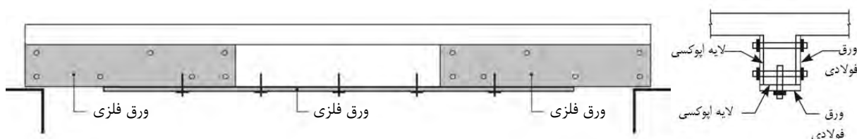
شکل ۶-۴-۲- تقویت خمشی و برشی تیرها با ورق فولادی
