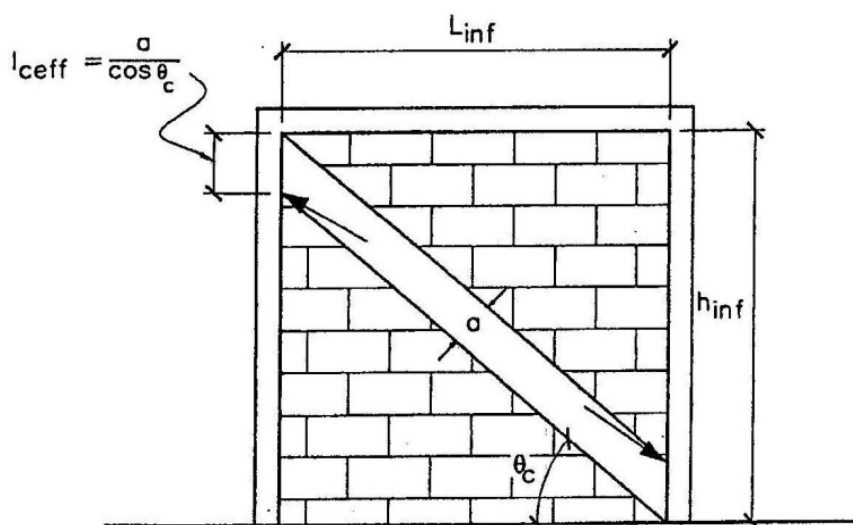
شکل مثال ۴-۲-ظ - نیروی برشی وارد به ستون از طرف پانل میانقاب
